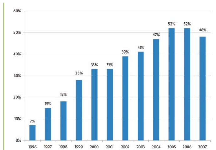
Emisiones de CO 2 de España desde la firma del Protocolo de Kyoto
